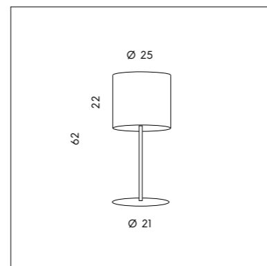
LT 1/503 1 x max 46W E27 CE IP20 □ ▽
