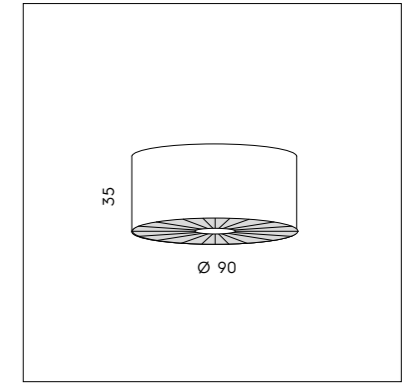
LS P/503-F 3 x max 46W E27 CE IP20 ▽
