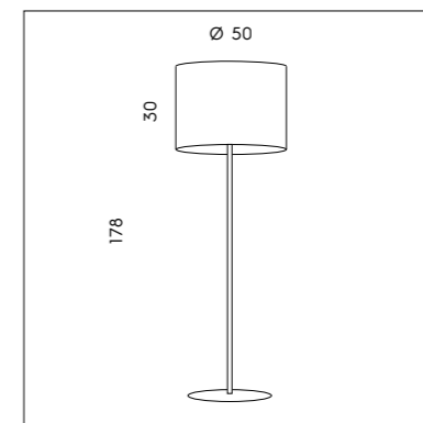
PI 3/503 1 x max 77W E27 CE IP20 □ ▽
