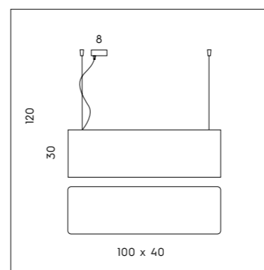
SP 8/501 3 x max 77W E27 CE IP20
