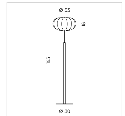
PI 3/332 1 x max 77W E27 CE IP20
