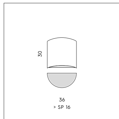
LP 6/503 1 x max 46W E27 CE IP20 ▽
