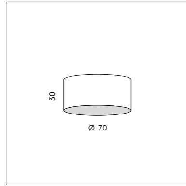
LS 5/503-L 3 x max 46W E27 CE IP20 ▽
