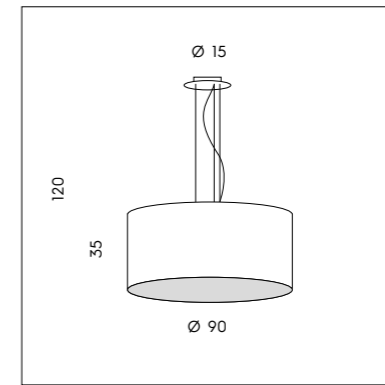
SP S/503-L 3 x max 77W E27 CE IP20 ▽
