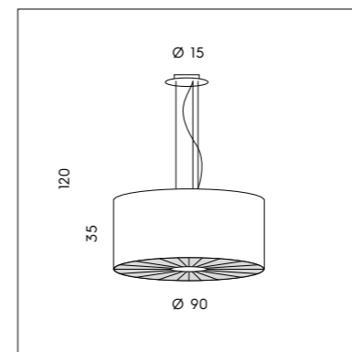
SP S/503-F 3 x max 77W E27 CE IP20 ▽
