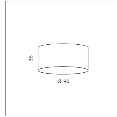
LS P/503 3 x max 46W E27 CE IP20 ▽
