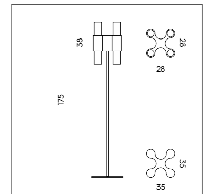
PI 3/331 8 x max 46W E14 CE IP20
